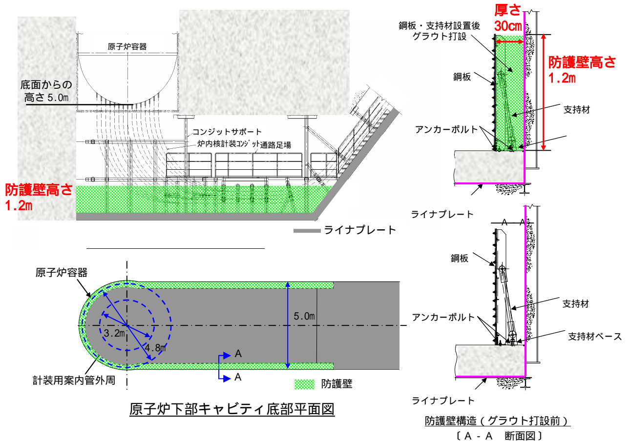
図 4.3.1 防護壁構造図 (断面図及び平面図)
